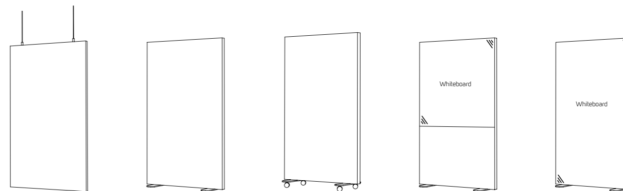
Hangend met spanners
